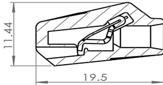
剖面 B-B
